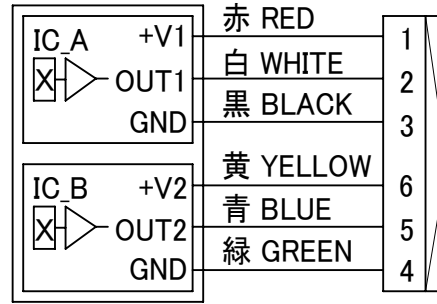
配線図 CIRCUIT DIAGRAM
