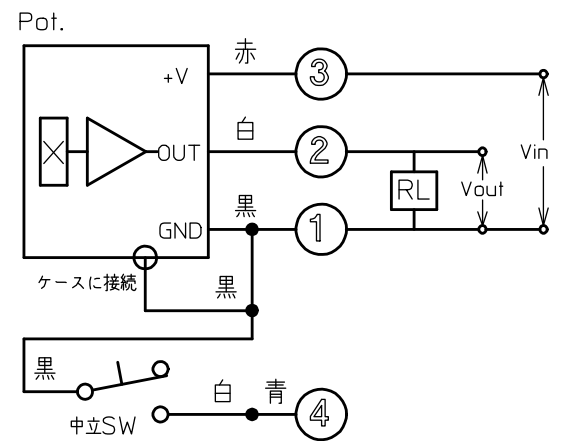
結線図
