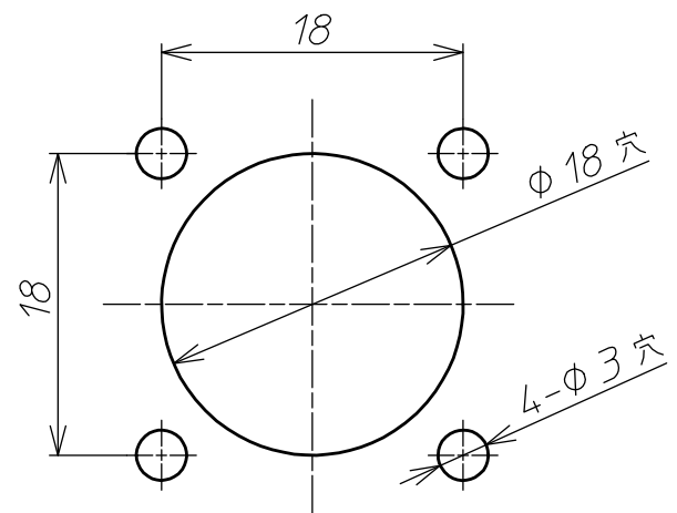
パネル取付面加工寸法図
